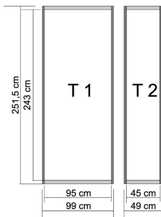
ТАБЛА//PANELS
