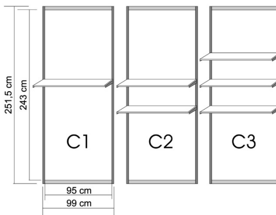
ЛАВИЦА//SHELF
