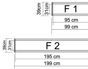
ФРИЗ//FRONT PANELS
